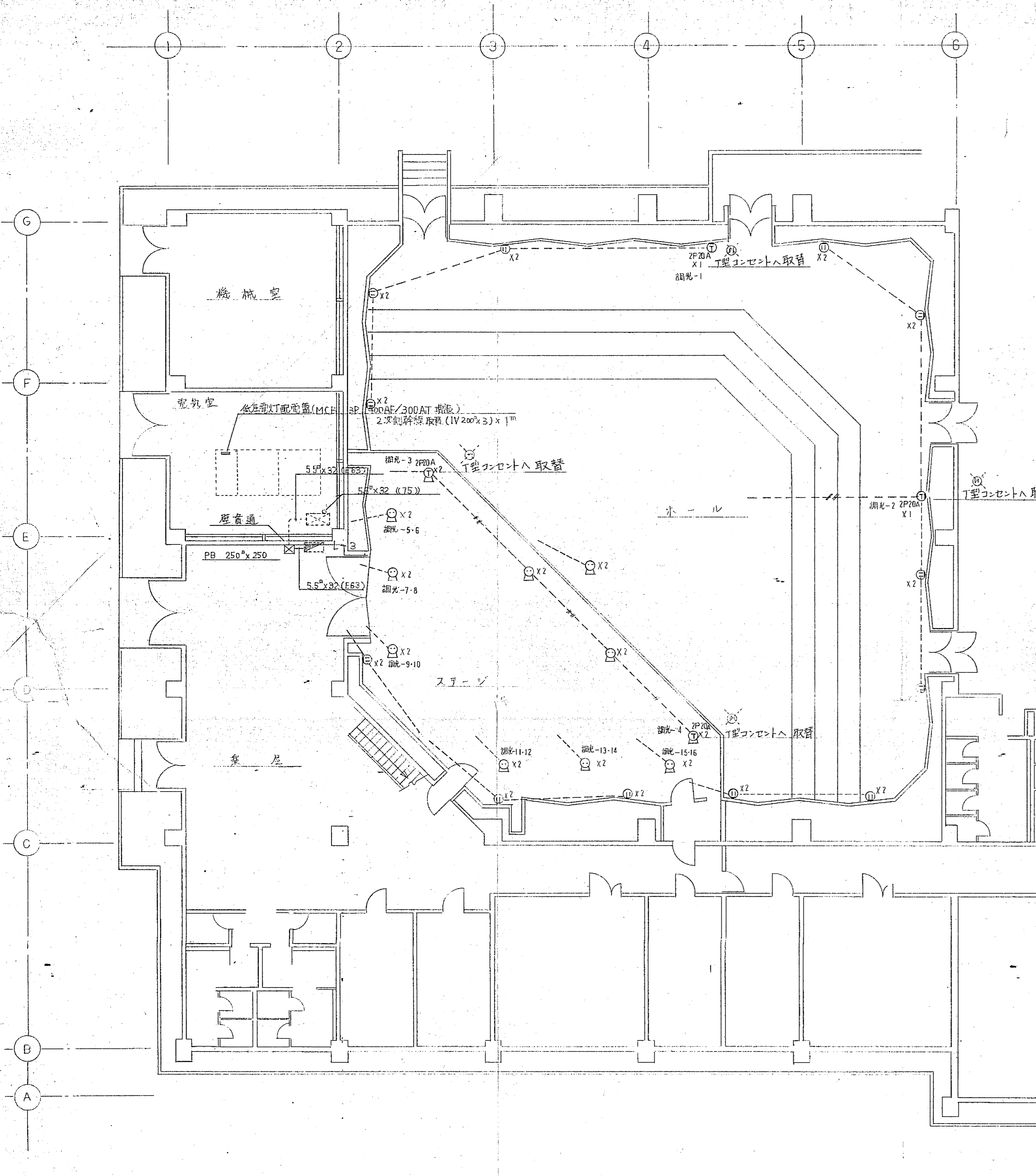
1階 調光設備配線図 s 1/100
