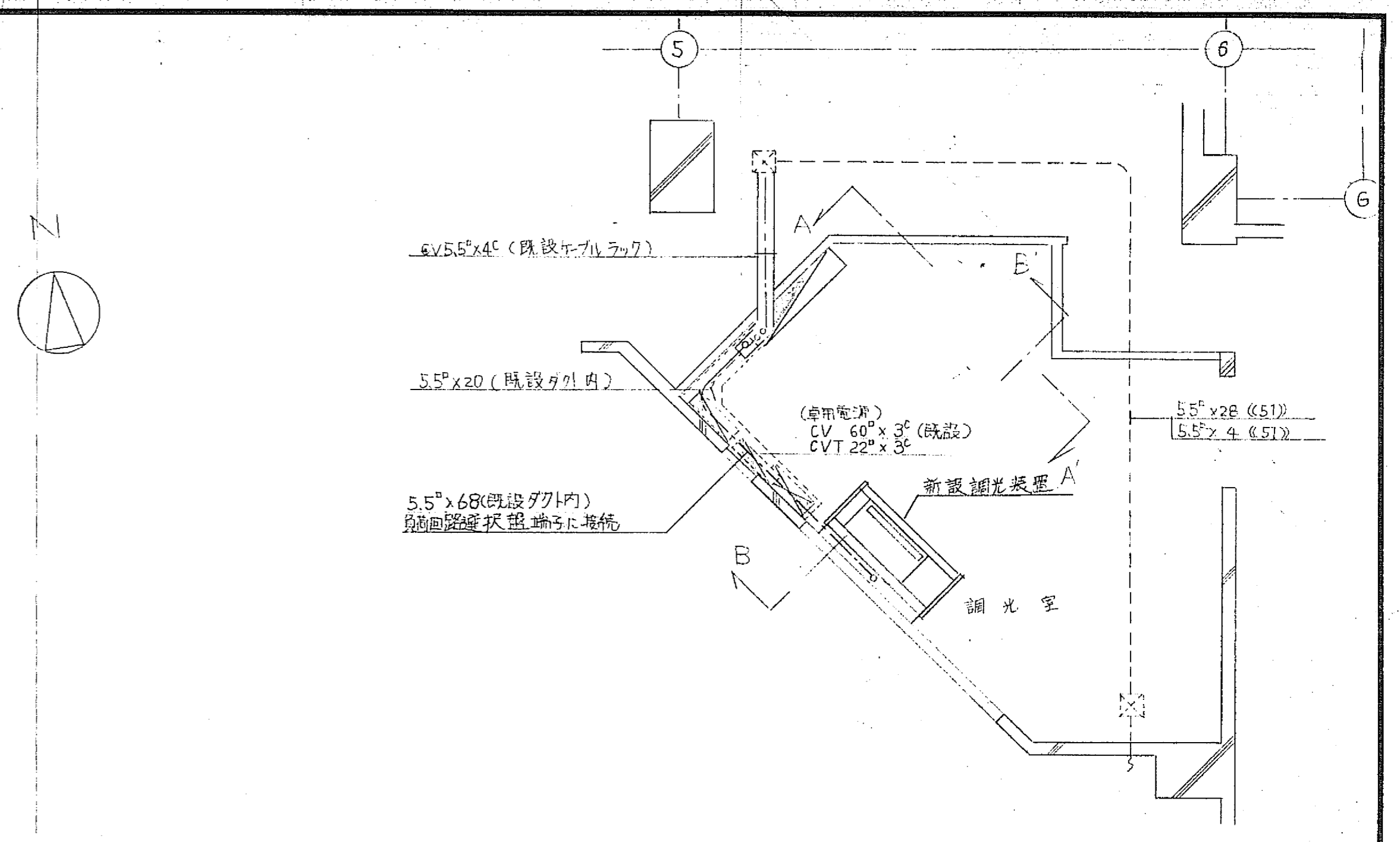
調光室配線図 5 1/50
