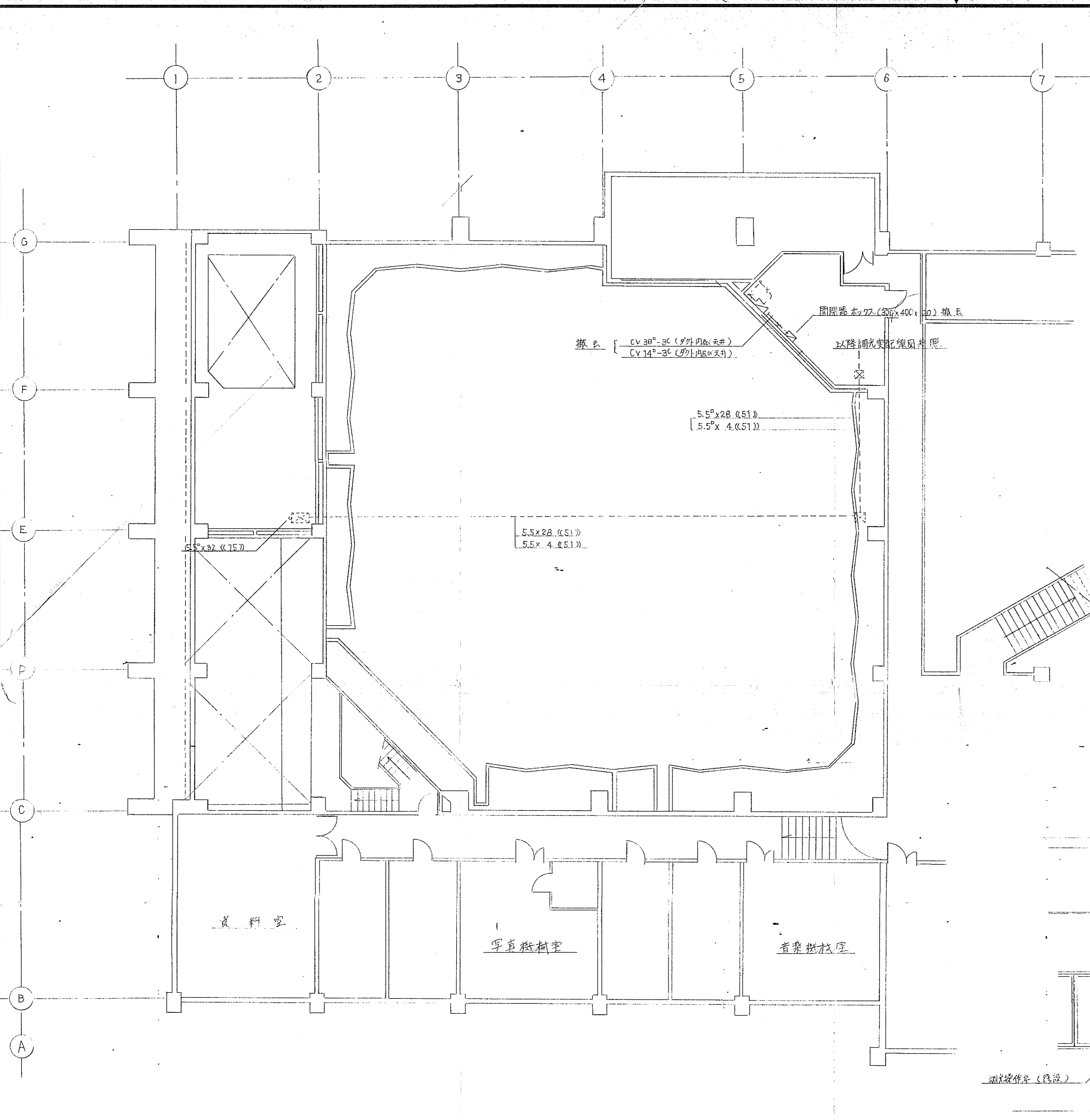
2階 調光設備配線図 5 1/100
